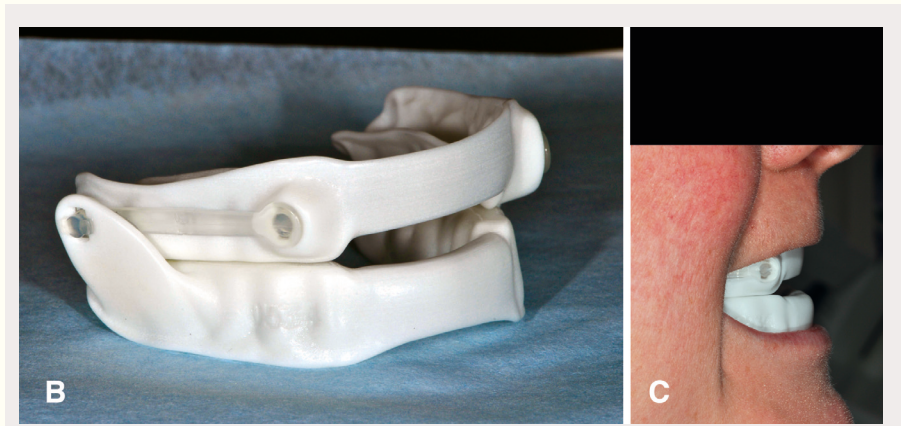
Figur 1B–C. Narval CC® søvnapnéskinne.
